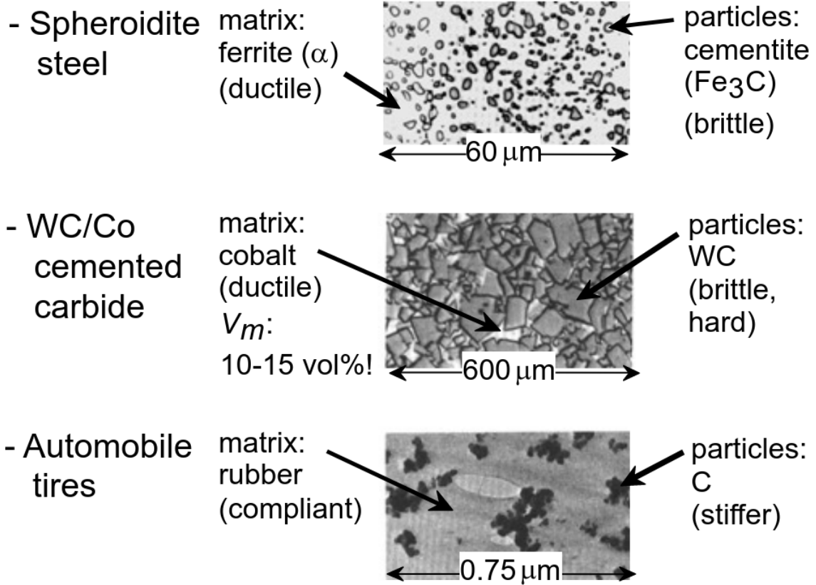
Slika 3: Uporaba ojačitve kompozitnih materialov z delci.
