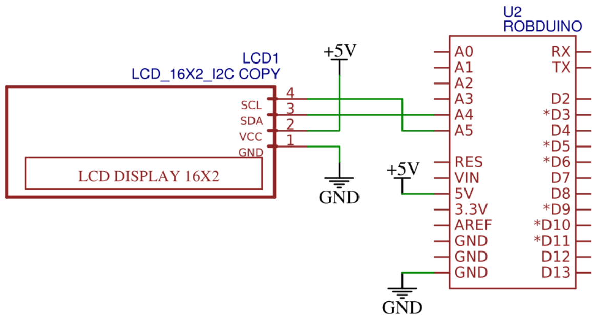
Figure 2.8: Povezava LCD na I2C vodilo krmilnika.
